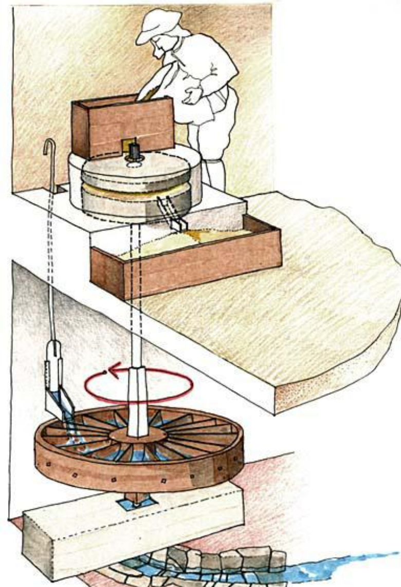
Esquema de funcionament d'un molí fariner tipus Font: Enciclopèdia Catalana
